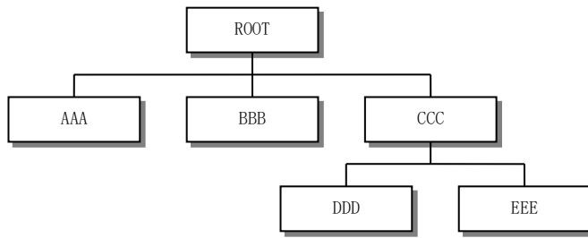
图 6-1 命令树结构
